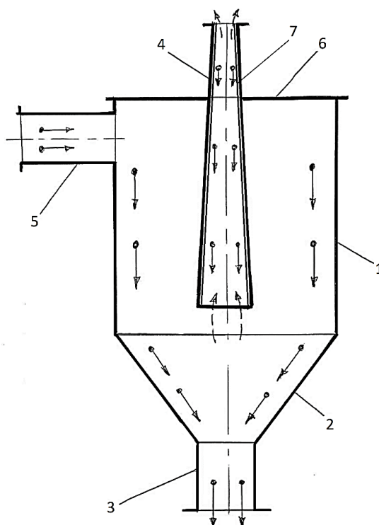
Рис. 1 – Схема циклона новой конструкции с повышенной степенью очистки дымовых газов от твердых частиц
