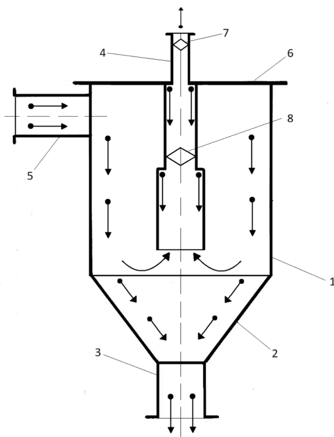
Рис. 1 – Схема новой конструкции эффективного фильтра-циклона с выхлопной трубой в виде цилиндра с диаметром, ступенчато уменьшающимся по высоте и дополнительной установкой фильтра на входе во вторую ступень
